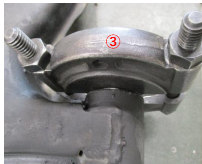
2. 起こしたブシュのフランジとロアアームの 間にベアリングリムバ③を取り付ける。
