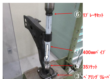
6. No.2ブシュはパイプ⑦を使って 抜く。
