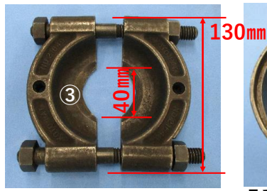
品番:09950-00020よりも 一回り小さいサイズのベアリングリムバ
