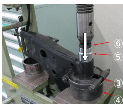
5. No.1ブシュを抜く。
