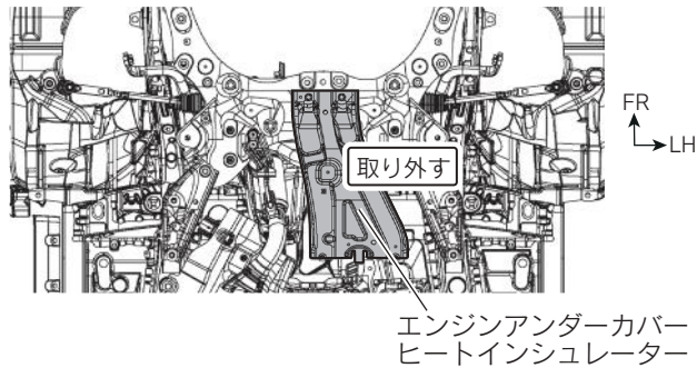
図2 下面視
