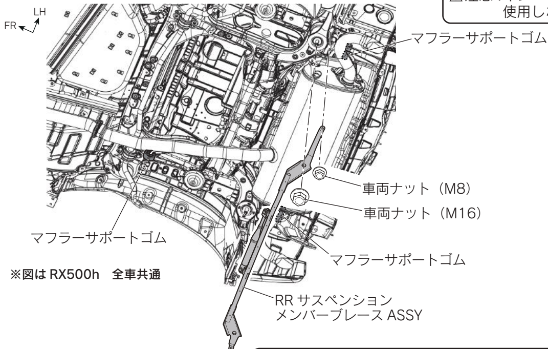
図 12 下面視 ※ L H 図示 左右共通作業
