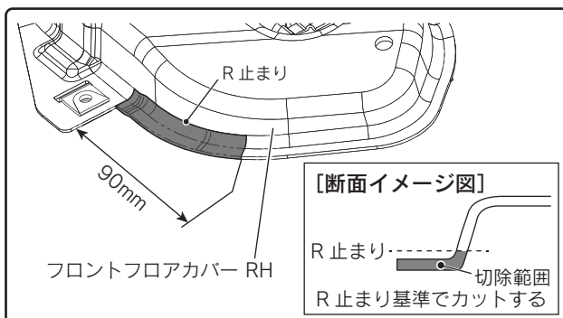
下面視
