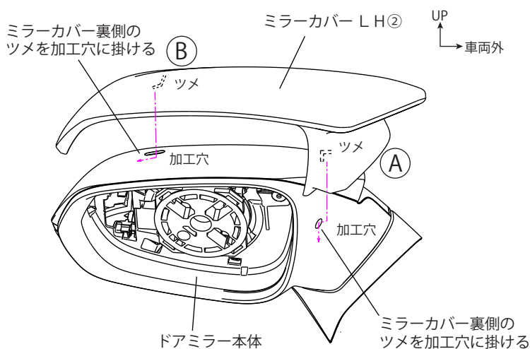
図8 ※LH図示 左右共通作業
