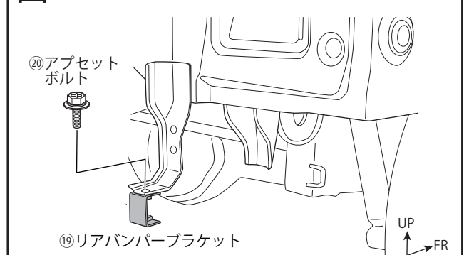
図4 ※左右共通作業（図はRH）
