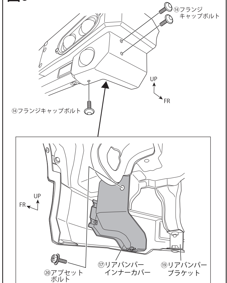
図6 ※左右共通作業（図はRH）
