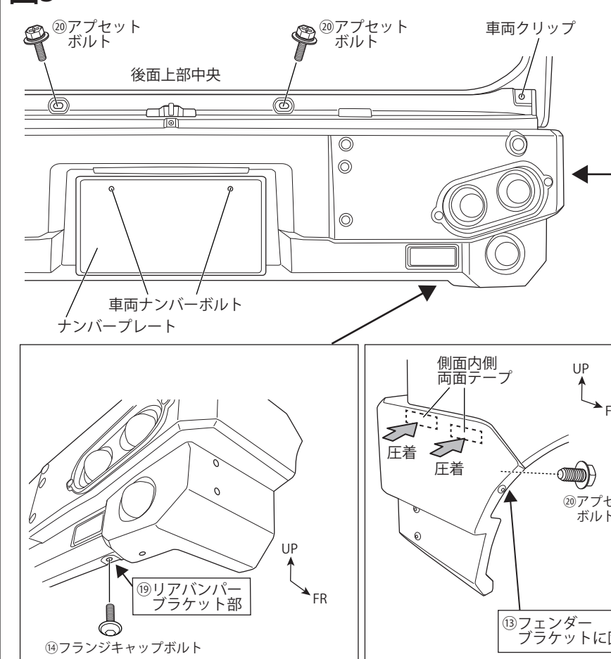
図5 ※左右共通作業（図はRH）
