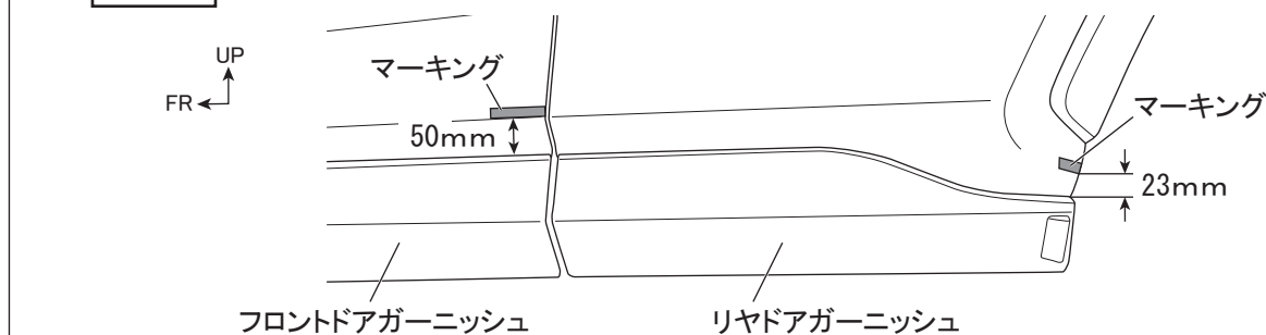
図6 側面視 ※LH図示 左右共通作業
