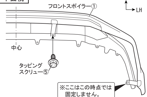
下面視
