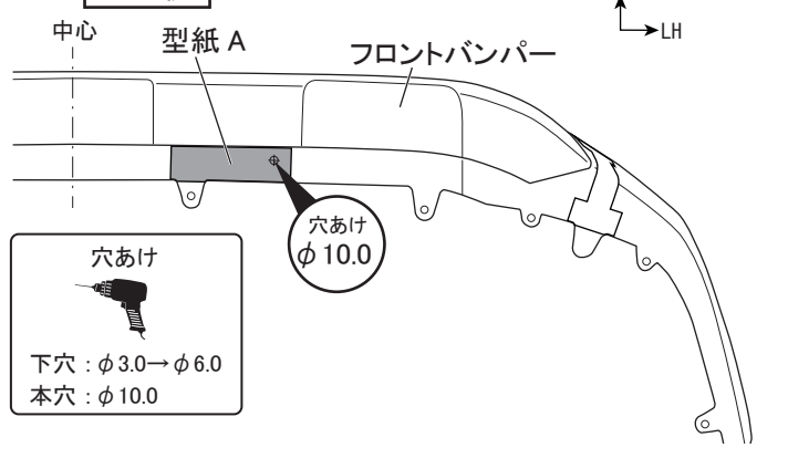
図 12 下面視 ※LH図示 左右共通作業
