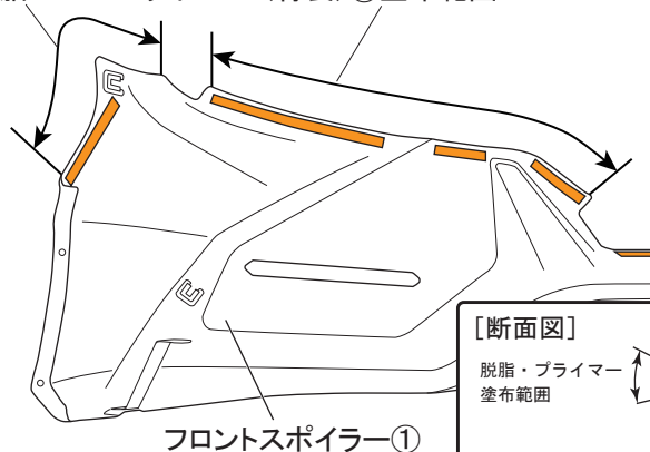
図3 裏面視 ※LH図示 左右共通作業
