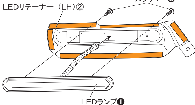
図 26 ※LH図示 左右共通作業
