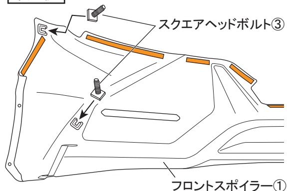
図 24 裏面視 ※LH図示 左右共通作業
