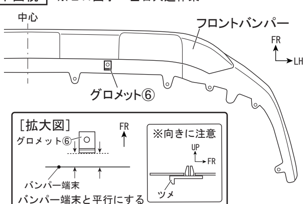
図 15 下面視 ※LH図示 左右共通作業
