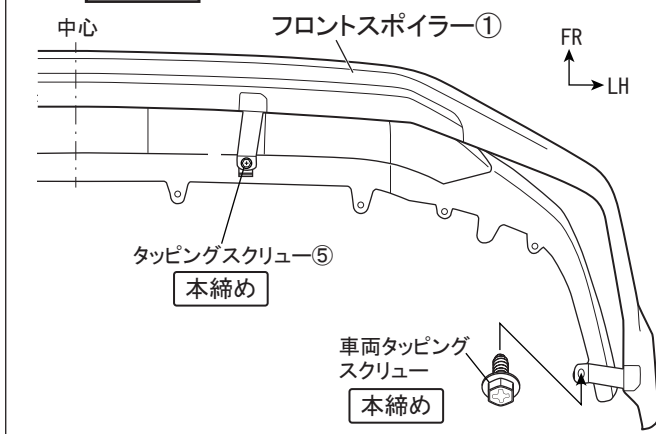
図 37 下面視 ※LH図示 左右共通作業
