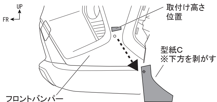
図 14 側面視 ※LH図示 左右共通作業
