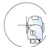
① 回転半径 895mm (脱着シートの後輪中心からの回転半径)
