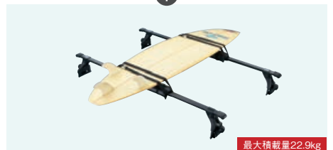
最大積載量22.9kg
