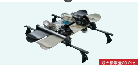
最大積載量20.2kg
