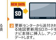
※写真はイメージです。
